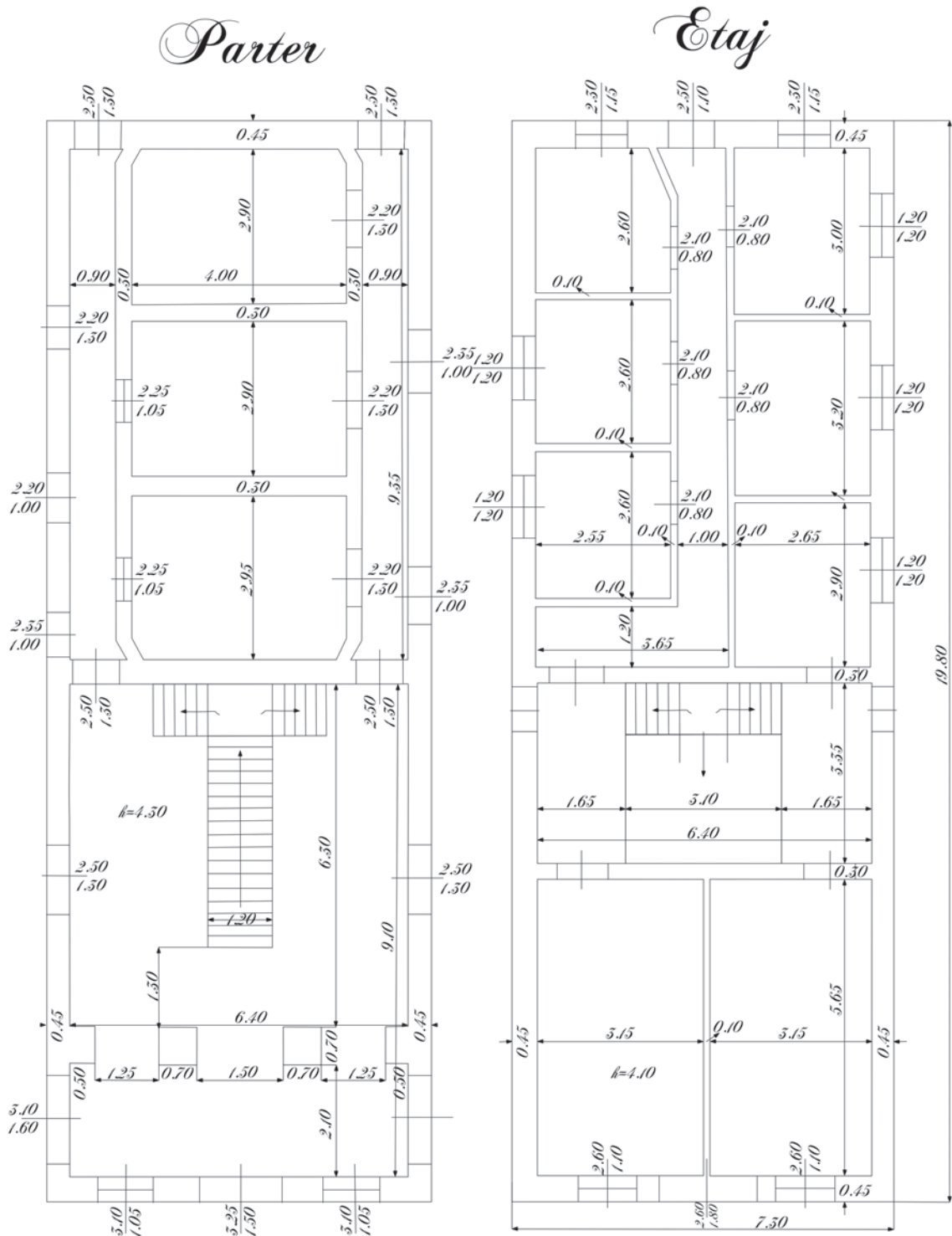
Fig. 33. Casa Cuza-Vodă din Galați, plan detaliu, parter zona centrală și etaj, realizat de ing. T. Popescu, 1937 (redesenat de Tudor Mandache, Muzeul de Istorie „Paul Păltănea” Galați).
